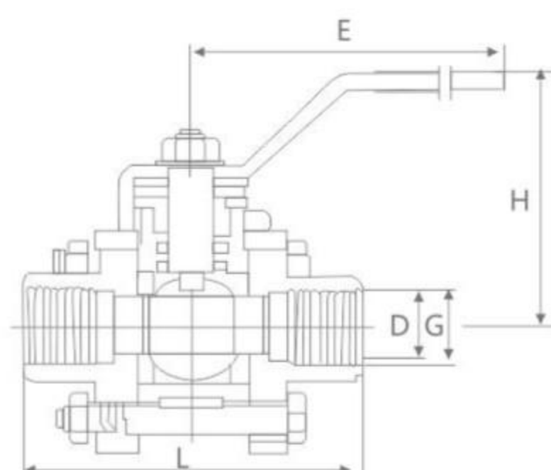
3PC Ball valve 三片式球阀
